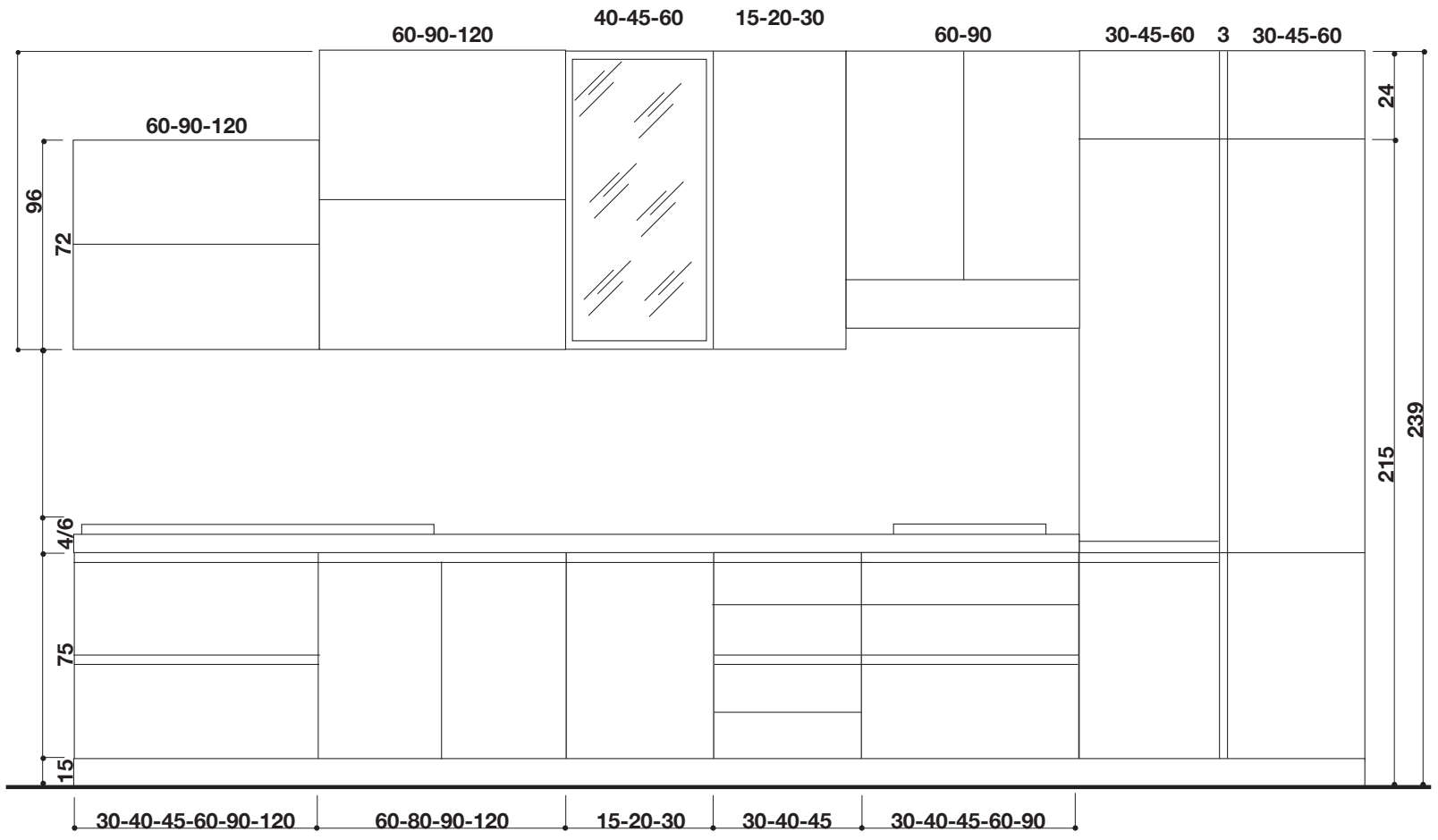
VISTA FRONTALE FRONT VIEW VUE DE FACE
