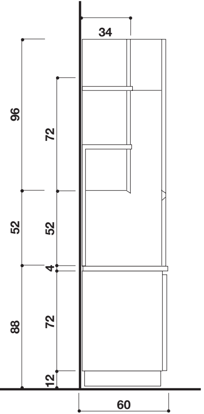
VISTA LATERALE SIDE VIEW VUE LATÉRALE
